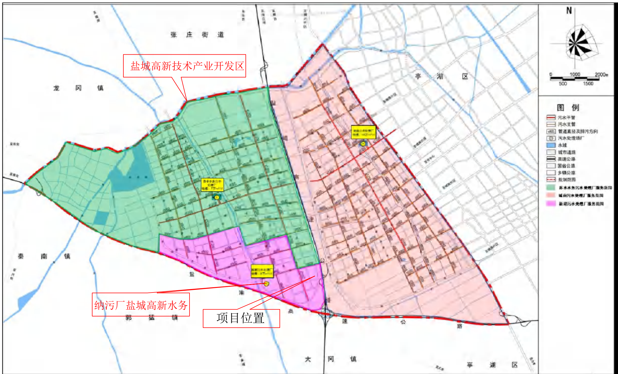
附图5 园区污水管网规划图
