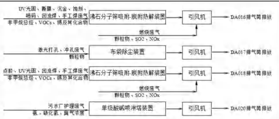
图 2-5 废气处理工艺流程图
