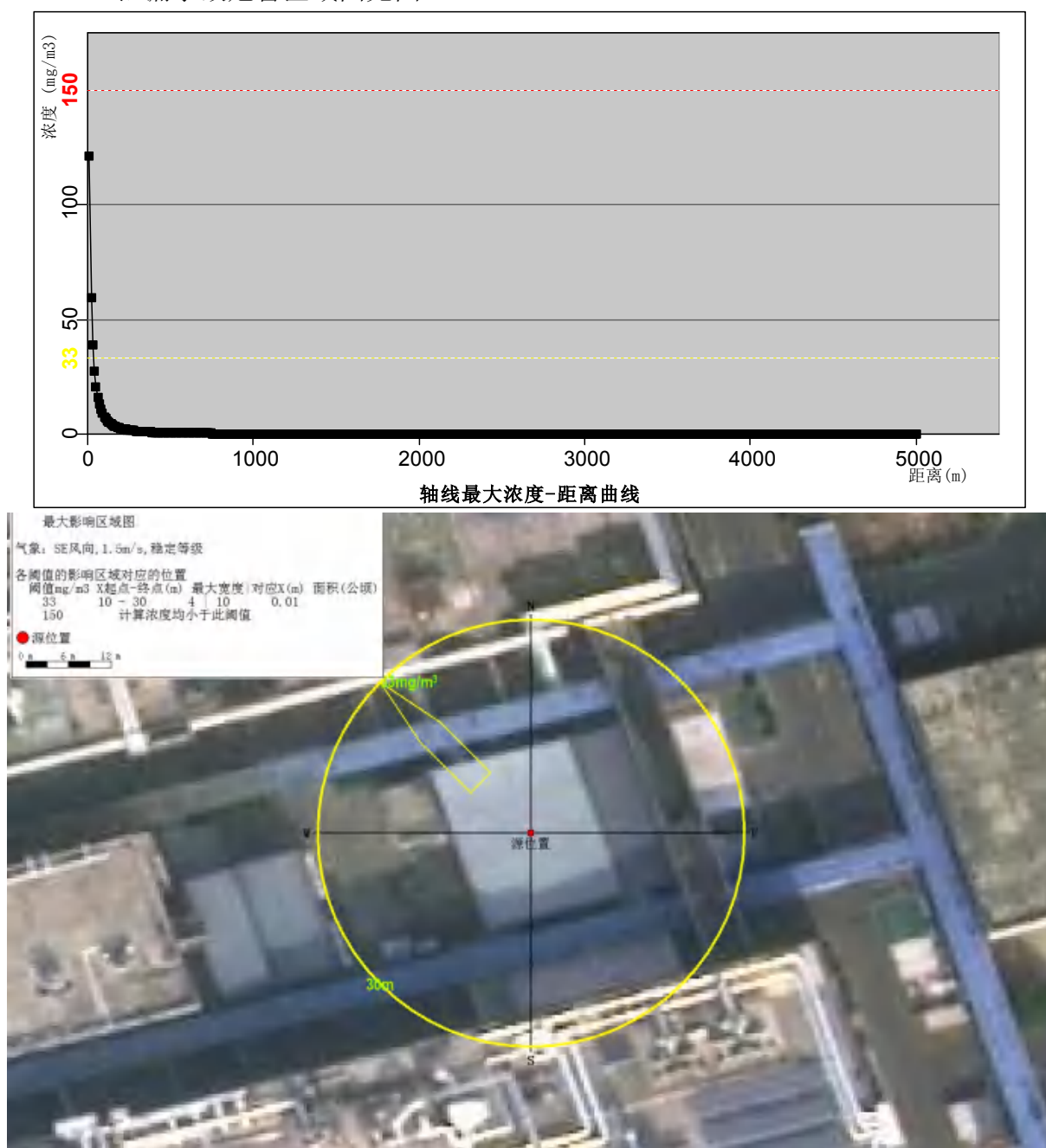
图 4-1 盐酸泄漏事故危害区域图
