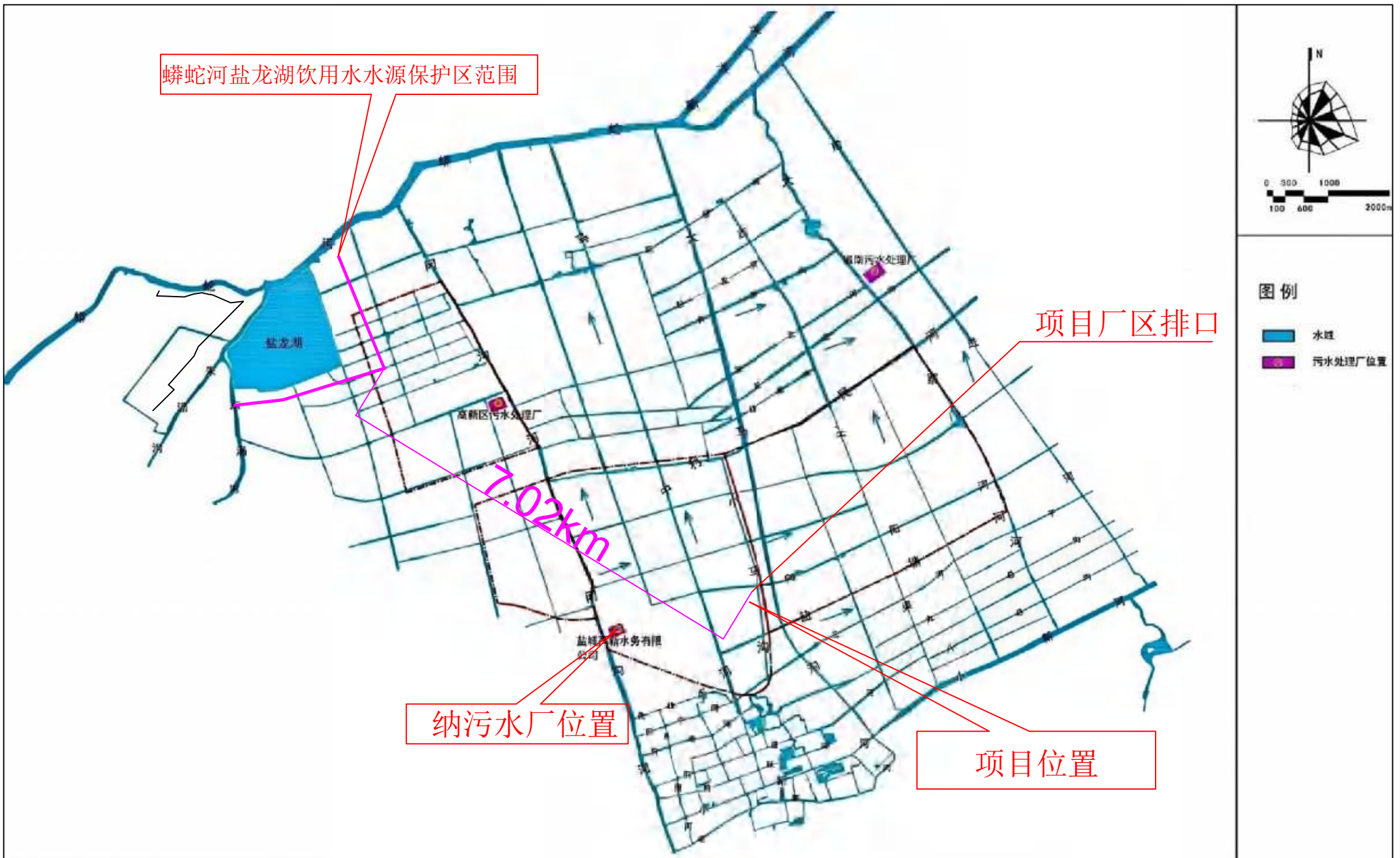
附图17 项目所在区域水系图
