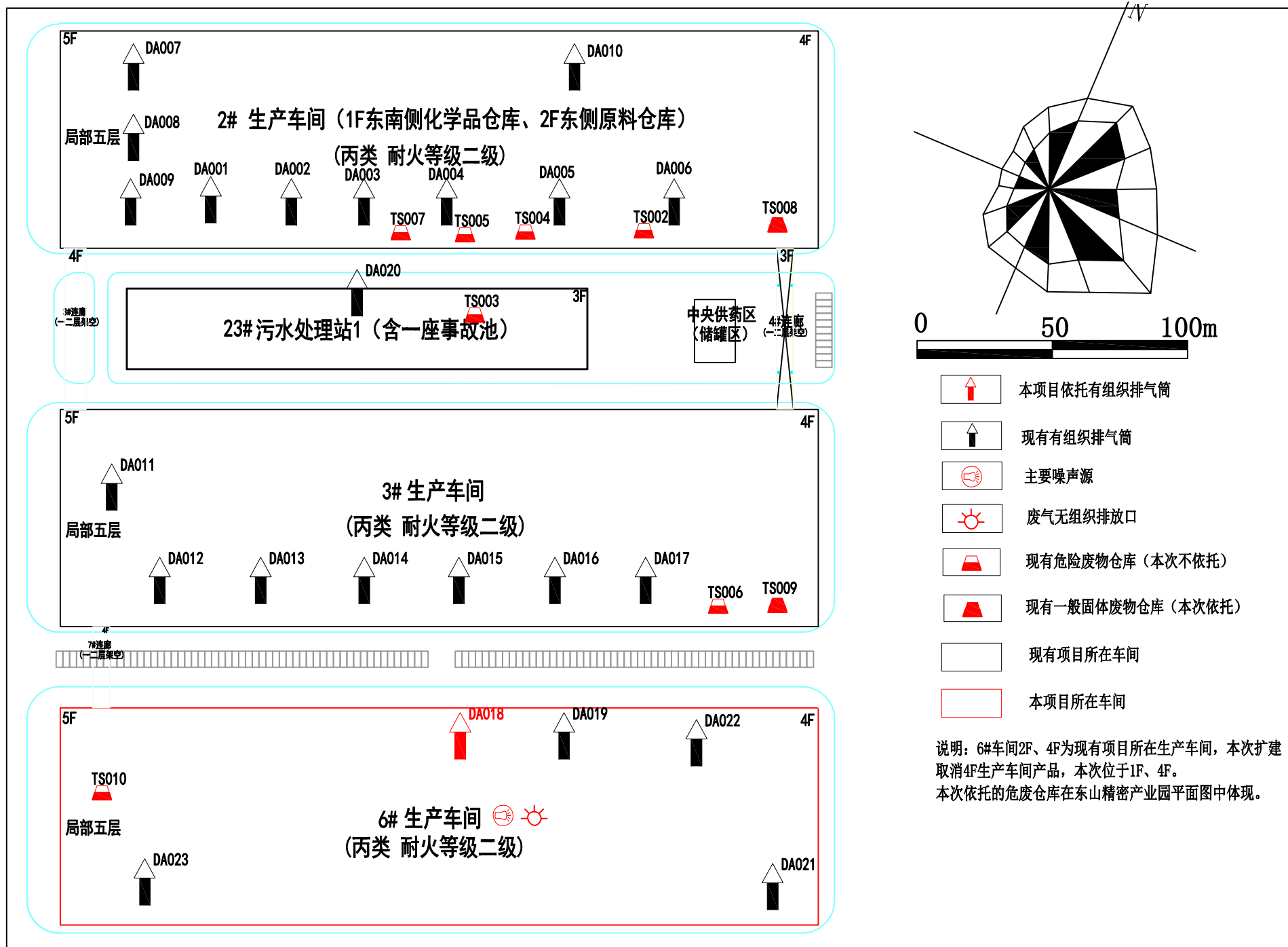
附图14 维信平面布置图
