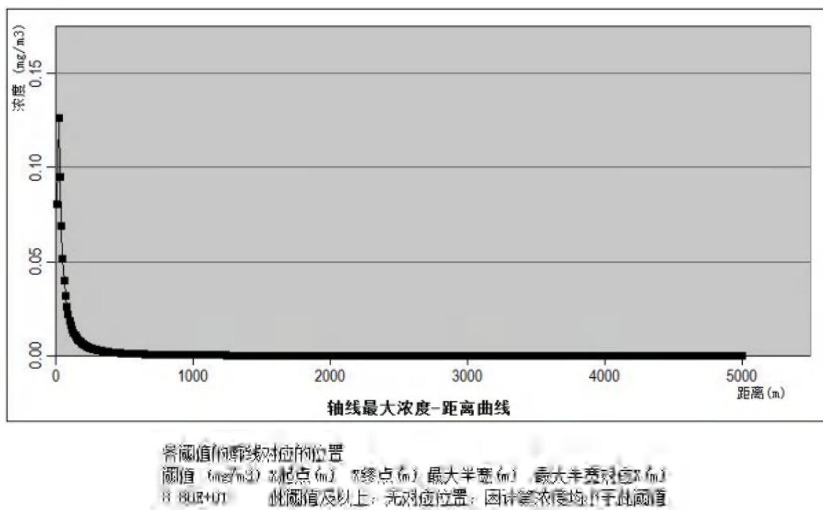
图 4-3 苯酚事故危害区域图
