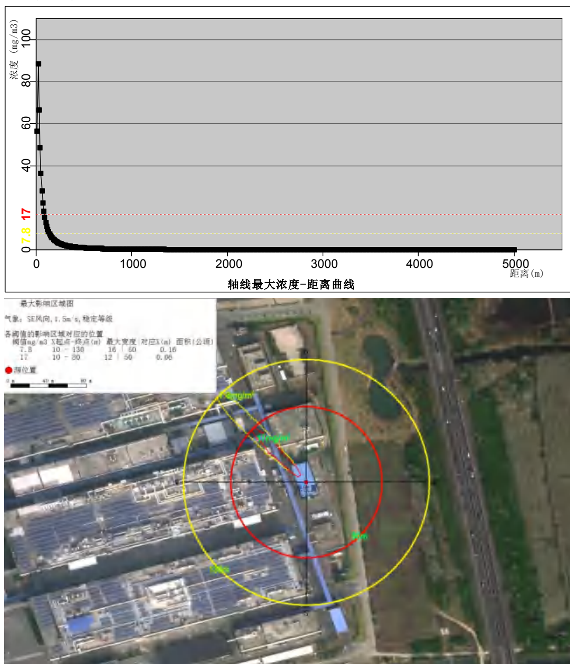
图 4-2 氰化氢事故危害区域图
