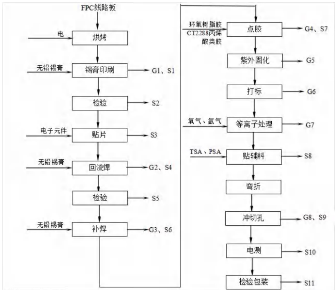
图 2-2 FPC 线路板生产工艺流程图
